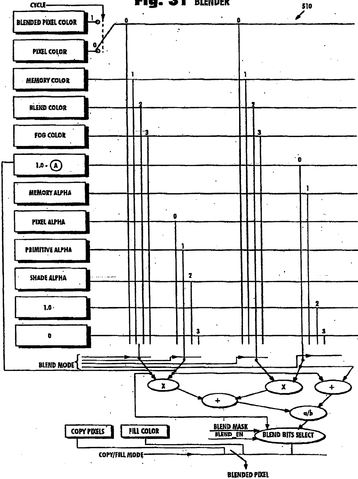
Fig. 31 BLENDER
